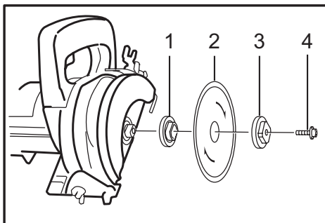
► 1. Brida interior 2. Disco de diamante 3. Brida exterior 4. Perno hexagonal de la cabeza de conexión
