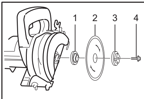
► 1. Bague interne 2. Meule diamantée 3. Bague externe 4. Boulon à tête creuse hexagonale
