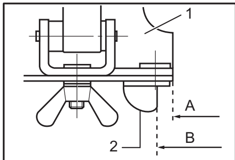
► 1. Base 2. Top guide
